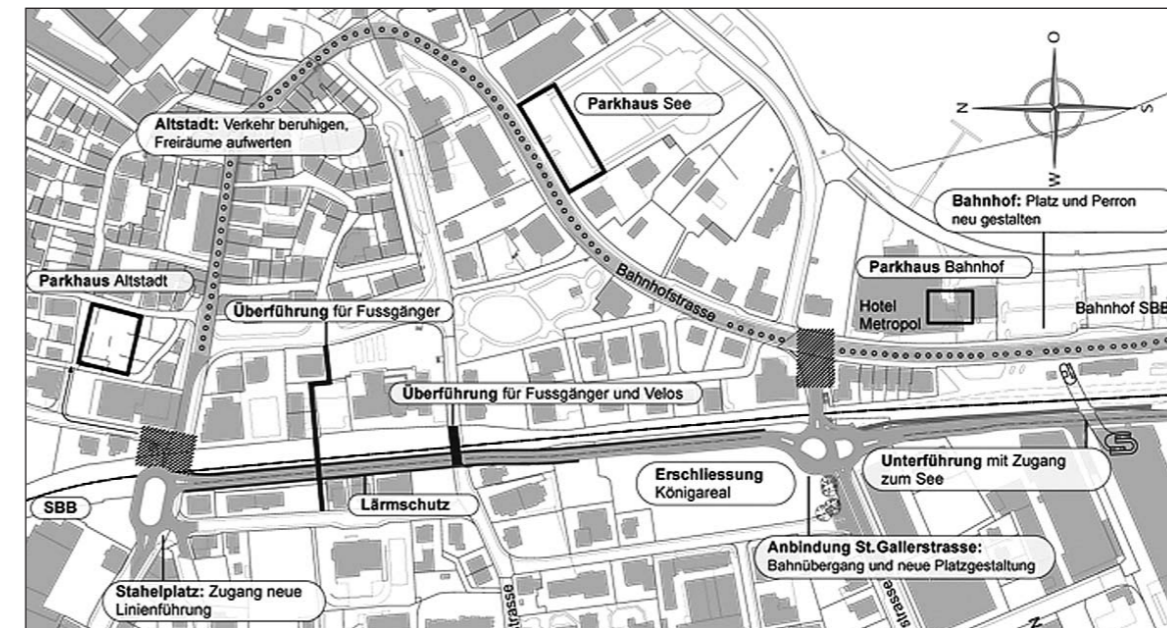
Die neue Linienführung der Kantonsstrasse K 148 ist das Schlüsselprojekt der Vision «Arbon 2020».
